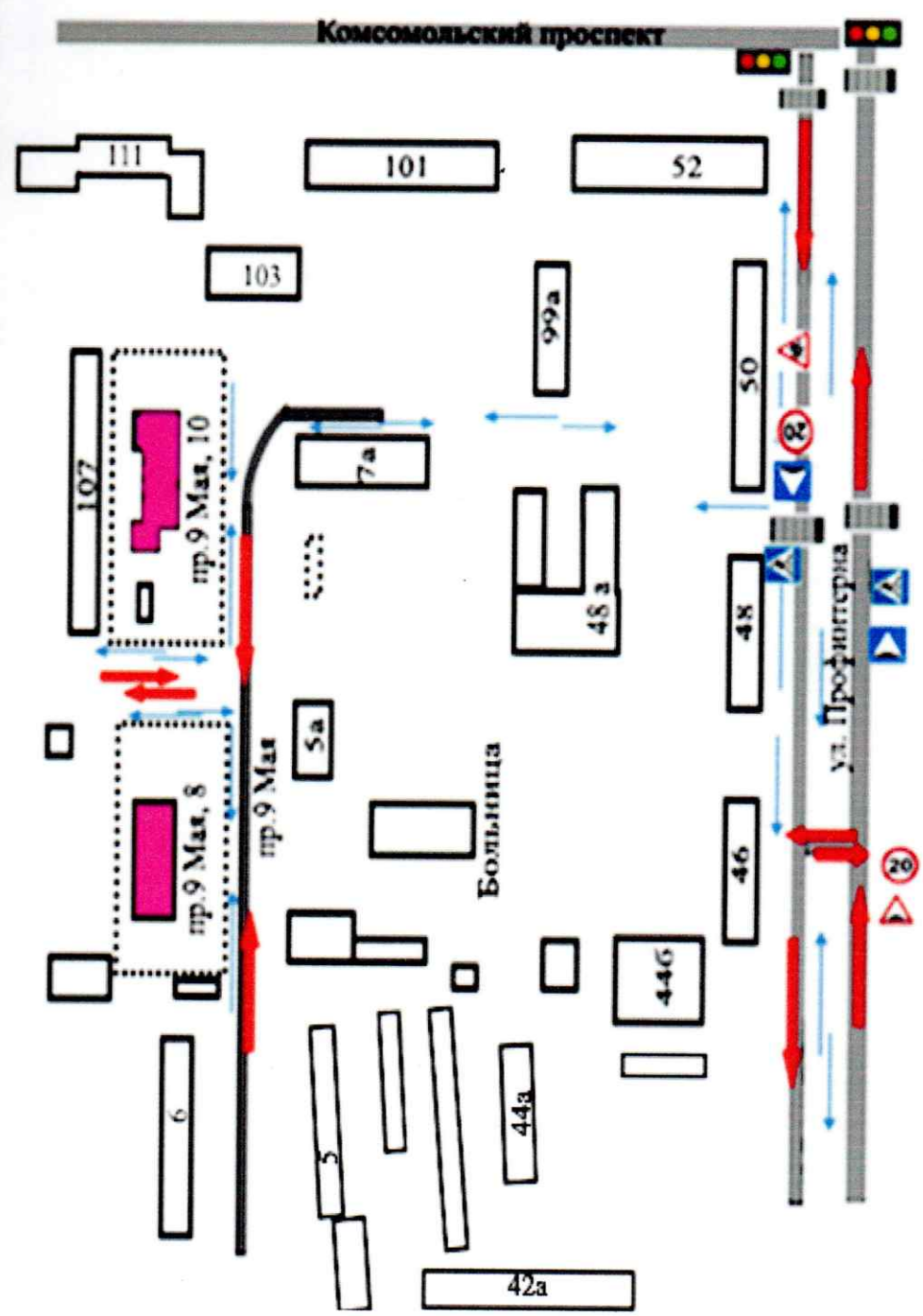
План-схема организации дорожного движения в районе МБДОУ «Детский сад №22» расположенного по адресу г. Барнаул, проезд 9 Мая, 10 (2 корпус).
